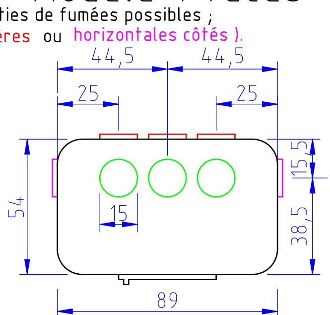
Modèle 4 faces
