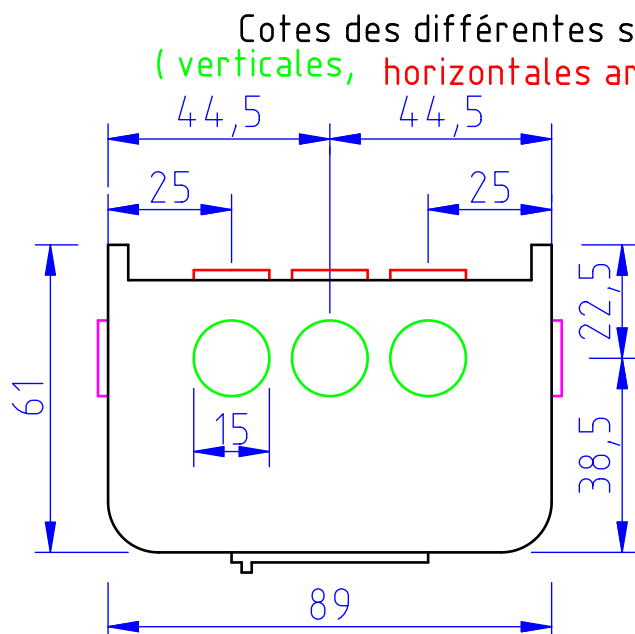
Modèle 3 faces
