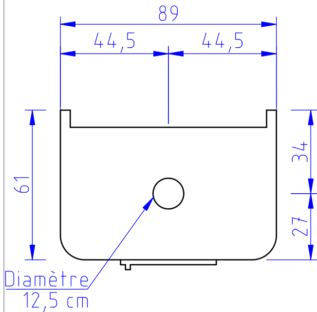
Modèle 3 faces
